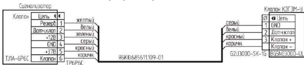
Рисунок В.1 – Схема подключения КЗГЭМ-У с разъемом BG5NO3000-UL
