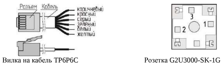
Рисунок В.3 – Схема подключения клапана КЗЭУГ с разъемом TJ1A-6P6C
